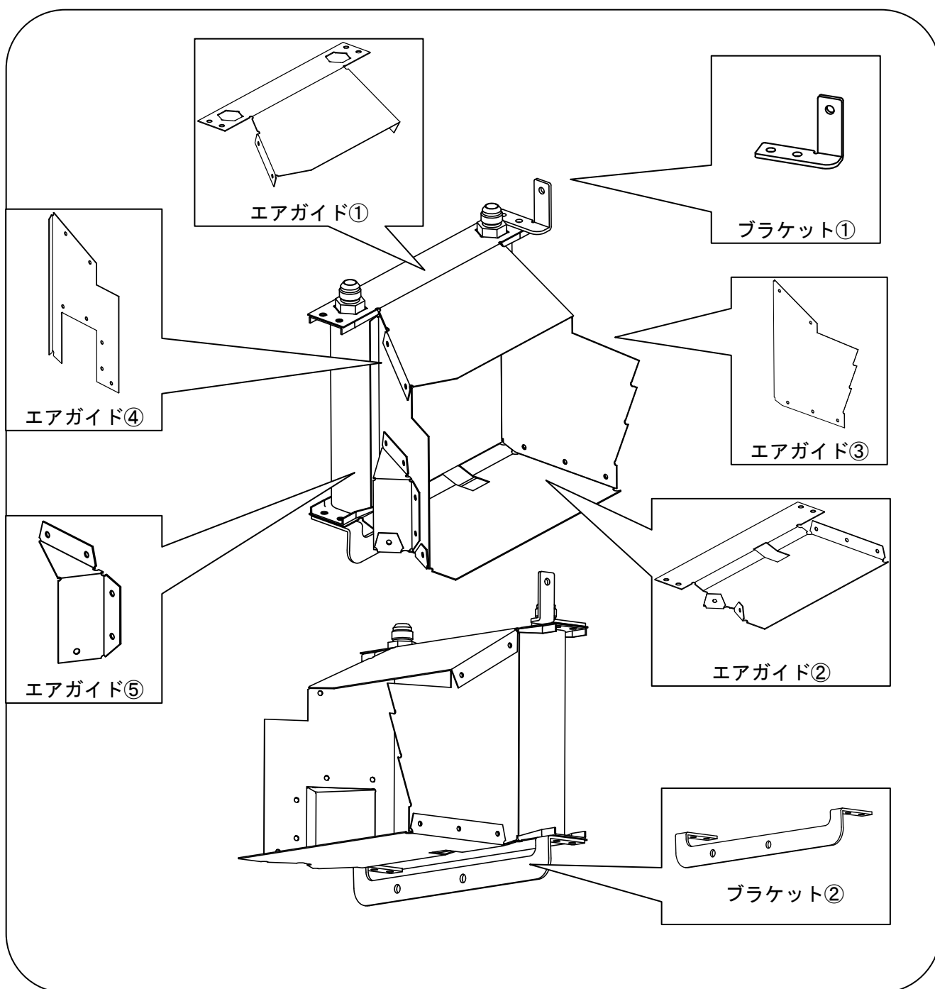
取付状態
