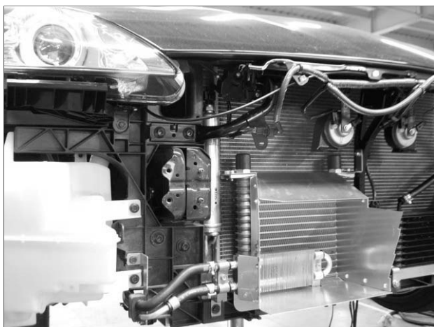
取付状態
